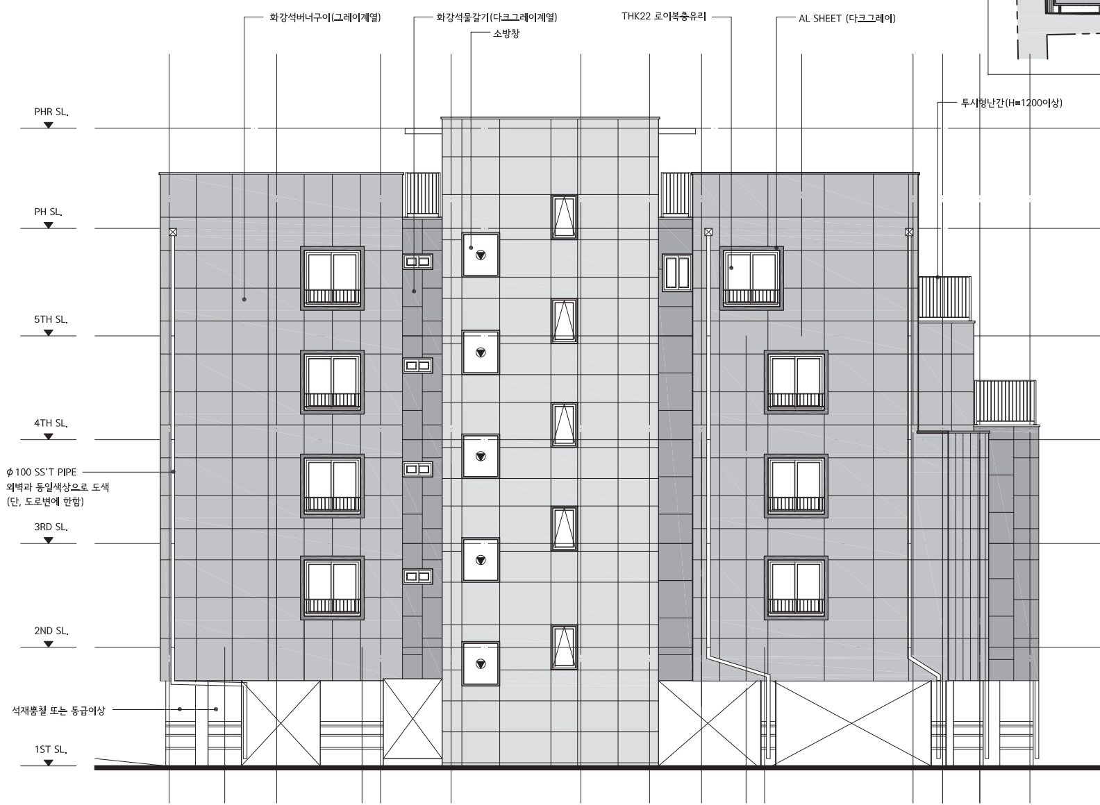
남 측 면 도 SCALE = 1/100
